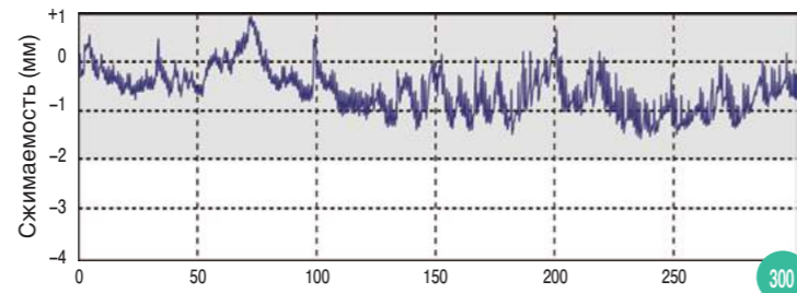
■ Изменение длины 16 мм сайдинга других производителей
