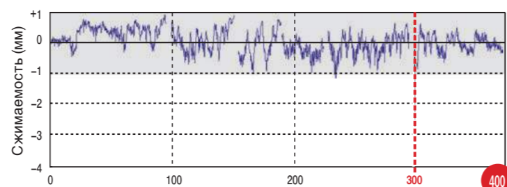
■ Изменение длины материала серии «Неорок»
